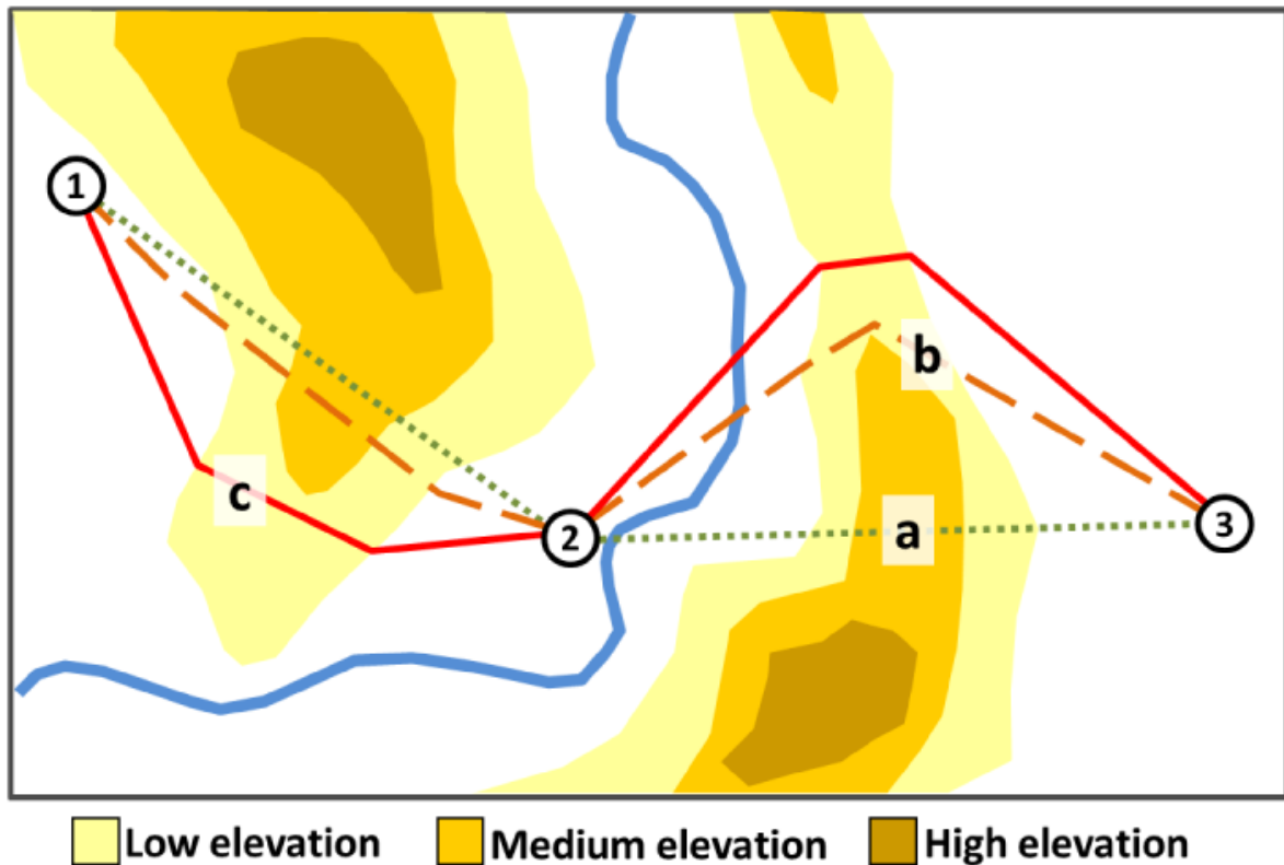
Figura 16: A influência do relevo nos traçados possíveis para um projeto geométrico de rodovia considerando o índice de desvio.
