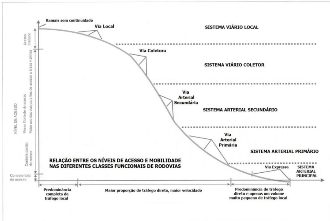
Figura 12: Classificação funcional das rodovias e relação entre mobilidade e acesso nos sistemas funcionais. Fonte: Brasil (1999).
