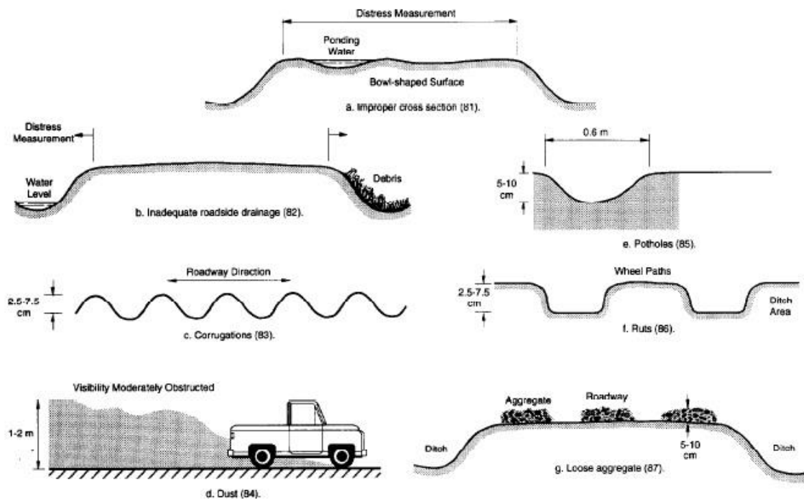
Figura 22: Defeitos comumente encontrados em estradas não pavimentadas. Fonte: Eaton e Beaucham (1995).
