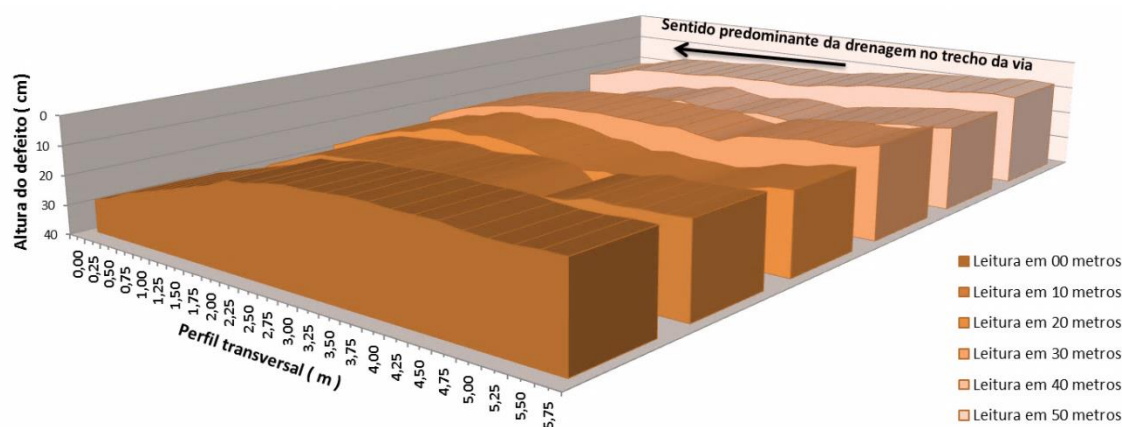
Gráfico 6: Perspectiva aproximada em 3 D das características dos defeitos no terraplino do trecho amostral 2AMD na rodovia que conecta a Vila de Cupixi à área de exploração mineral na serra do rio Vila Nova.
