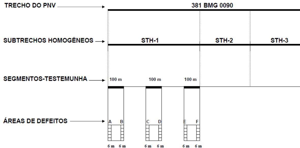
Figura 20: Esquema para escolha dos subtrechos amostrais para avaliação das condições físicas das rodovias federais.
