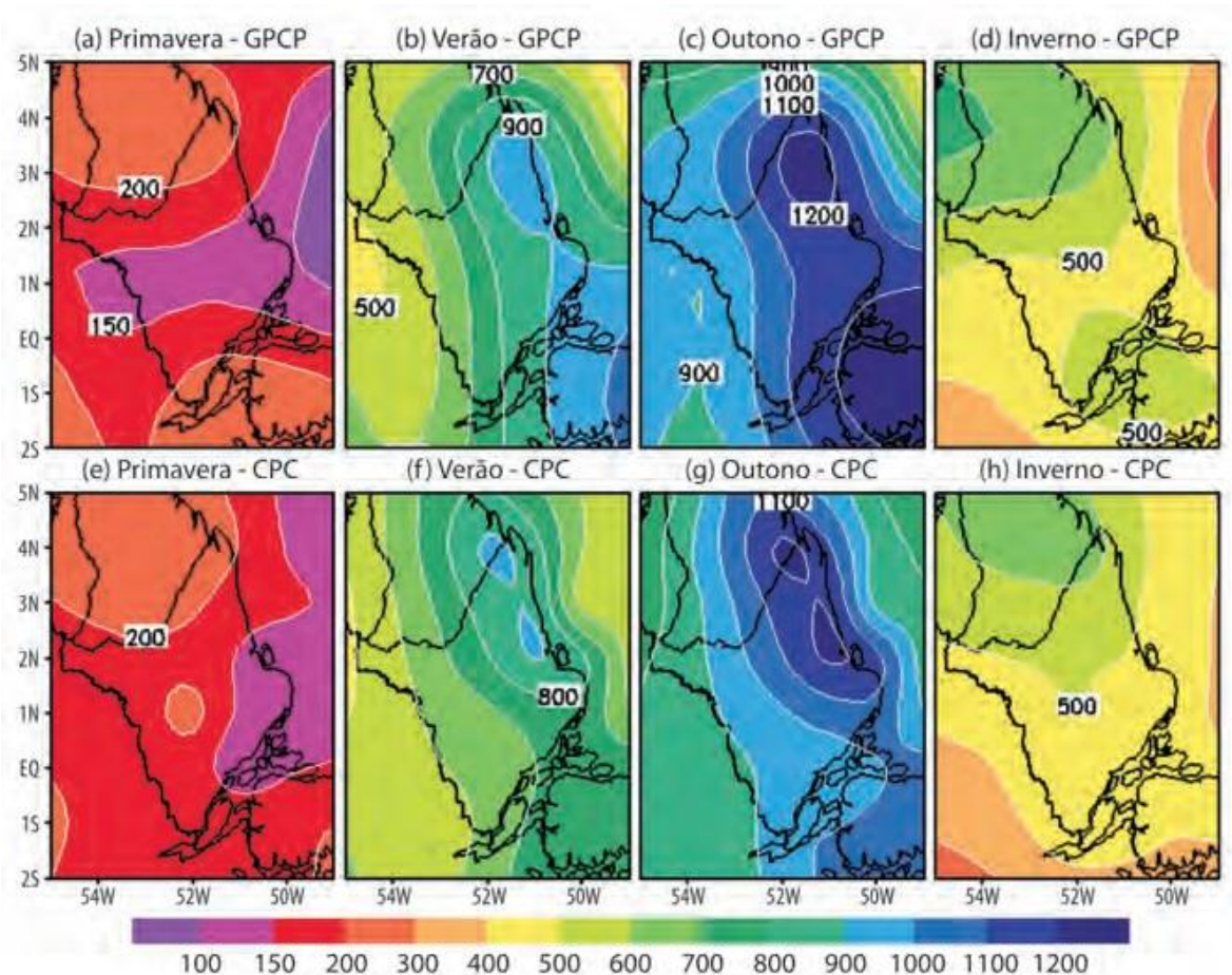
Figura 2. Mapas climatológicos da precipitação sazonal, em mm para o estado do Amapá (30 anos: 1978-2007) com dados do Centro de Previsão Climática (CPC) e do Global Precipitation Climatology Project (GPCP) Fonte: Cunha e Souza (2010)
