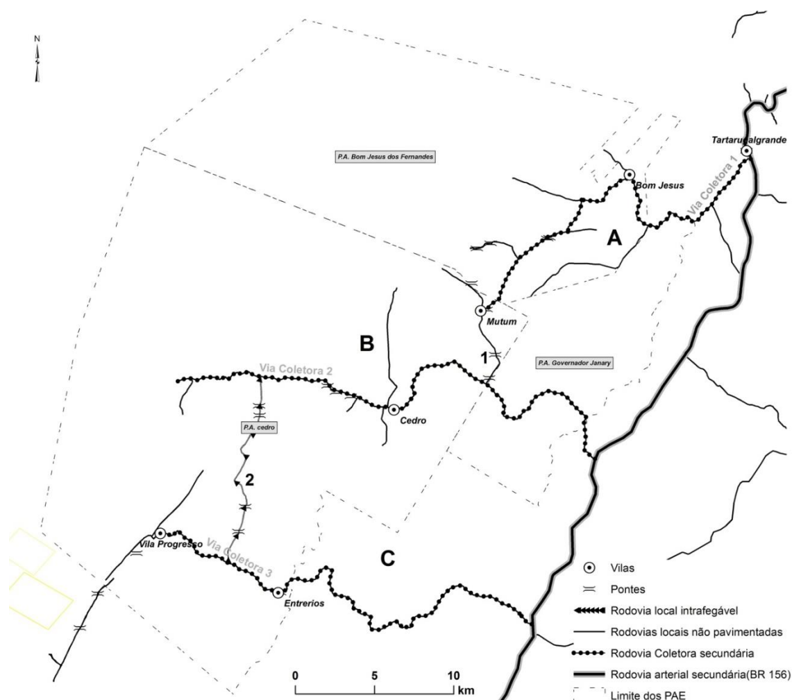
Figura 45: Topologia e classificação do sistema viário nos assentamentos Cedro, Bom Jesus dos Fernandes e Governador Janary.
