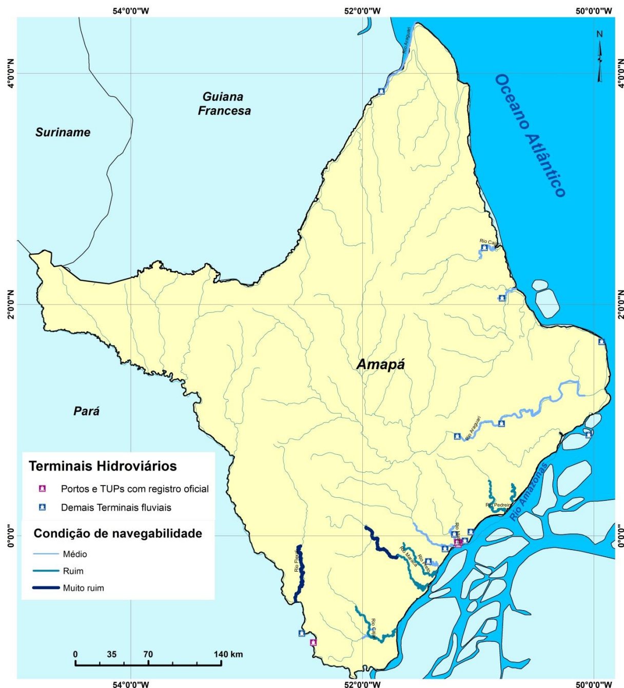
Figura 36: Identificação dos terminais hidroviários e caracterização da condição de navegabilidade nos rios com trechos navegáveis no Amapá.
